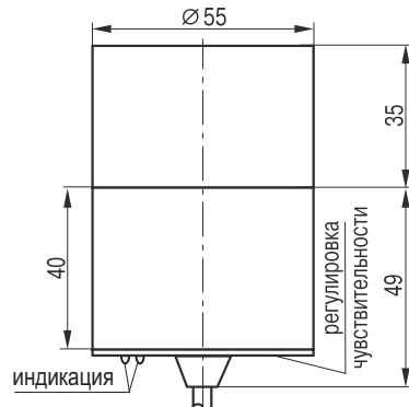
Габаритный чертёж
